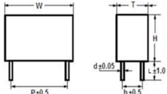
直脚 4 针脚型（4 pins）
